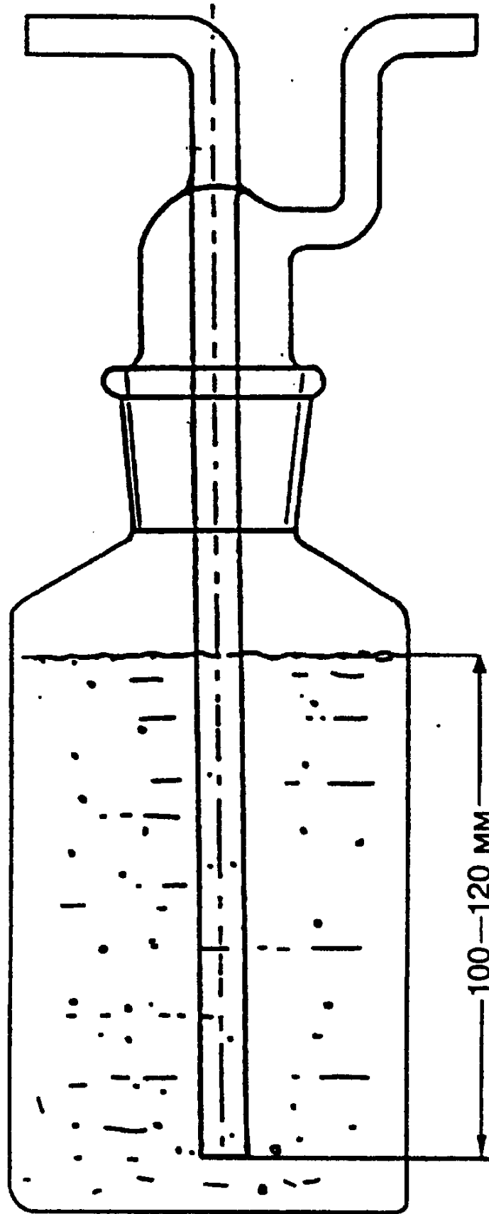
Рисунок 2 - Сосуд-смеситель
