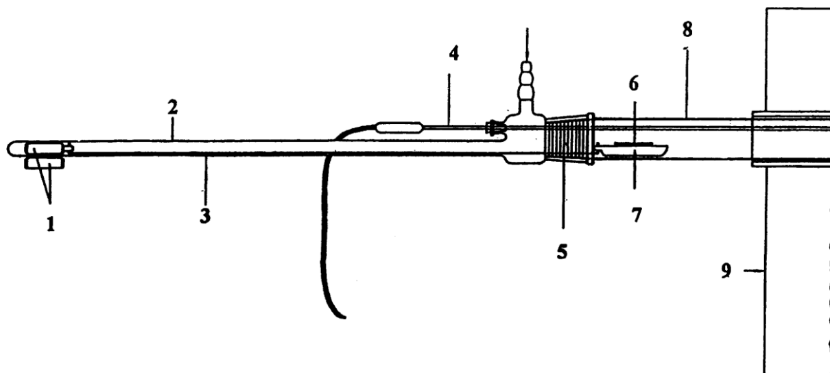
Рисунок 1 - Устрйоство для введения лодочки в зону нагрева трубчатой печи
